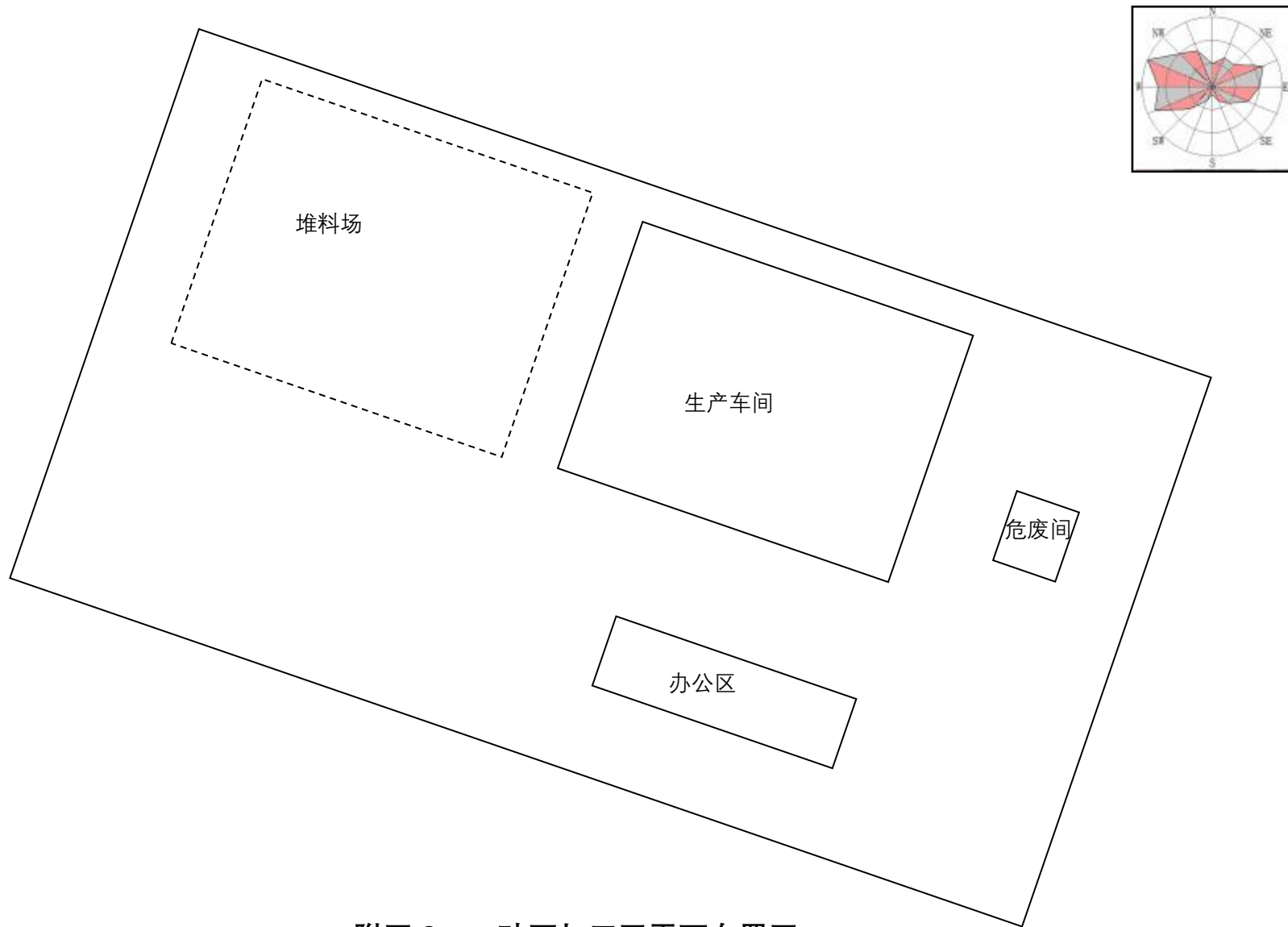
附图 3 砂石加工区平面布置图
